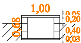
VISTA COM ATERRO ESCALA 1:50
